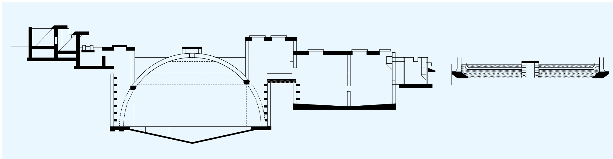
Figura 2. Plano da seção Chazanga FSTP com toma, BGD, tanque de sedimentação, câmara de expansão e filtro de cascalho 4 adaptados pelo SNV
