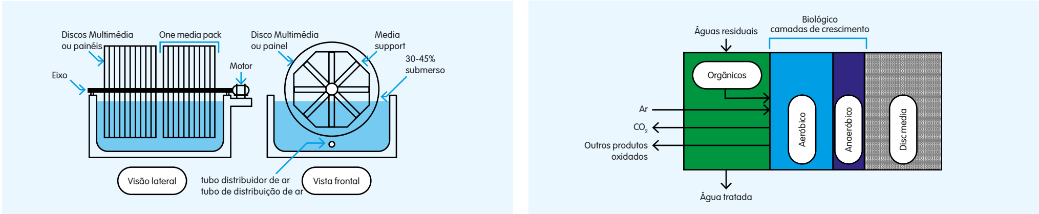
Figura 2. Diagrama esquemático de um RBC típico (esquerda) e uma seção transversal esquemática da face de contato do meio da cama em um RBC (direita), 3 adaptados por SNV
