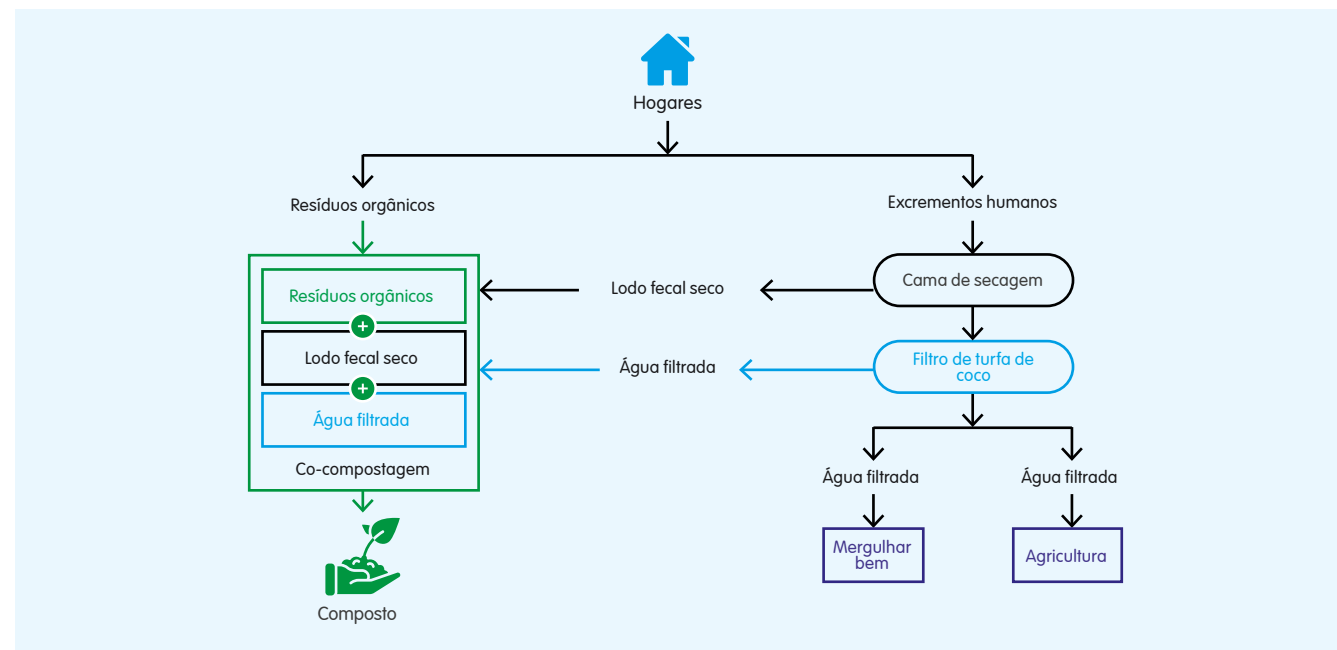
Figura 1. Diagrama de fluxo de tratamento, 1 adaptado pelo SNV
