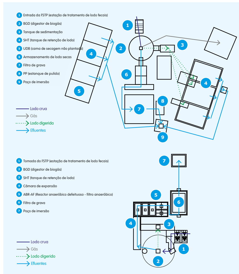
Figura 1. Apresentação do plano de distribuição e fluxograma de Chazanga FSTP (topo) 2 e do plano de distribuição e fluxograma de Kanyama FSTP (inferior) 3 adaptados pelo SNV
