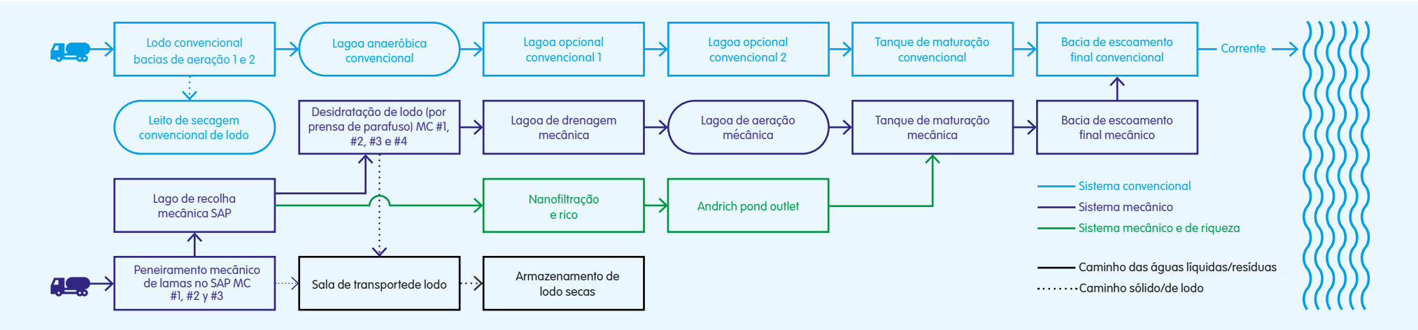
Figura 1. Fluxograma de blocos de Duri Kosambi FSTP 1
