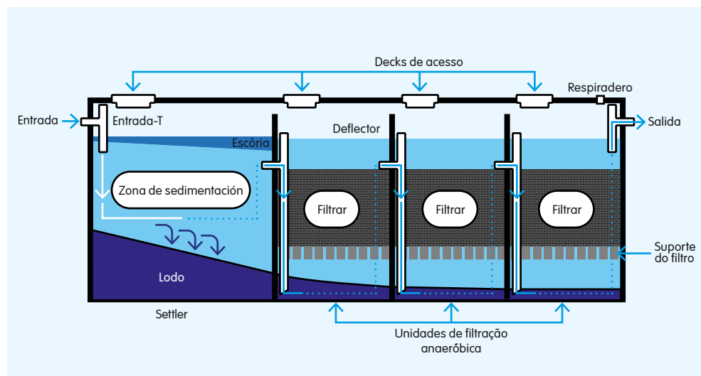
Figura 1. fluxograma de tratamento padrão DEWATS, 1 adaptado pela SNV
