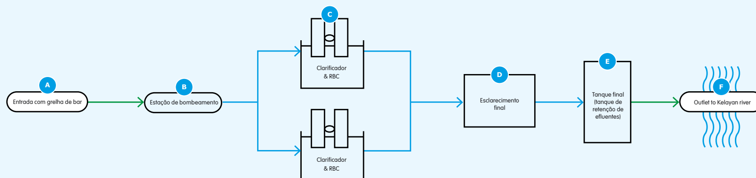
Figura 1. Processo de tratamento no Pekapuran Raya WWTP, 2 adaptado pelo SNV
